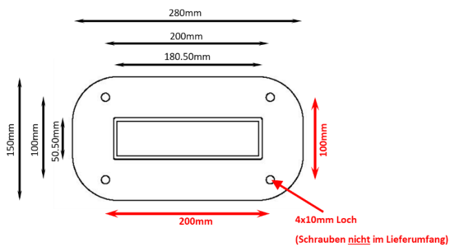
Grundplatte
